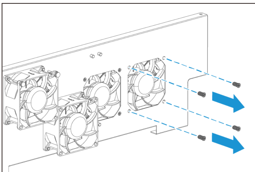
システムファン
