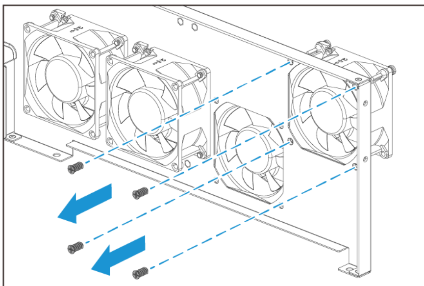
2.5 インチドライブベイファン
